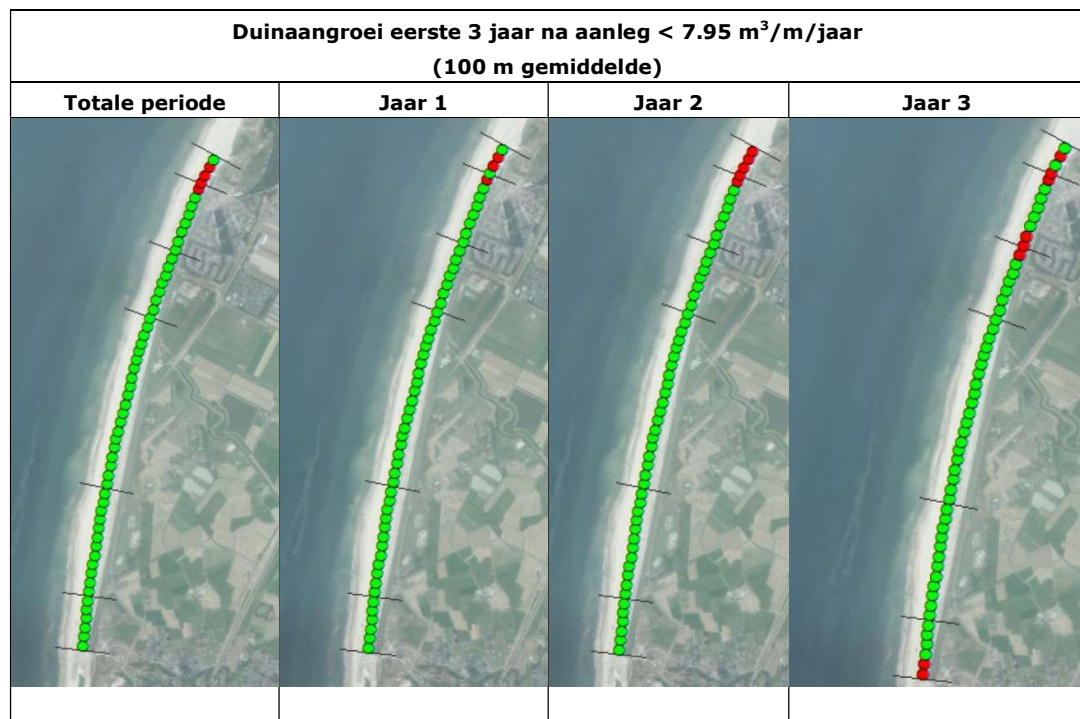
Figuur 4-4: Overzicht van locaties langs de HD waarbij de aanzanding meer (groen) en minder (rood) is dan 7,95 m 3 /m/jaar.
