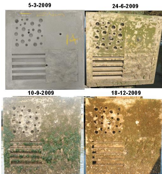
Figuur 3.10 De begroeiing van de ecobetonplaten aan de rechterbinnenzijde van palenpaar 2 van steiger 7 in de Scheurhaven in de loop van 2009.
