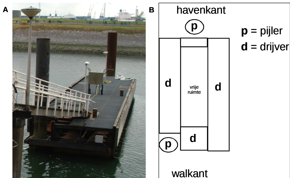
Figuur 2.8 A Het uit aparte drijvers opgebouwde ponton aan steiger 3 in de Scheurhaven B Schematisch overzicht van dit ponton
